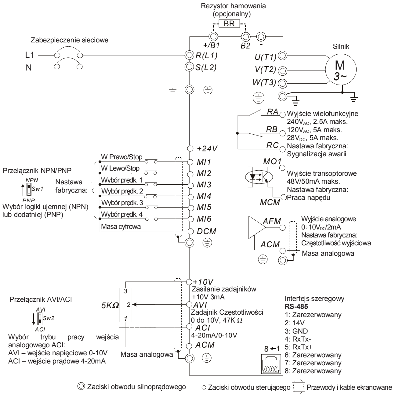
Rysunek 3 - dotyczy następujących napędów rodziny AMD-E: AMD-E 0007/RN21, AMD-E 0011/RN21
